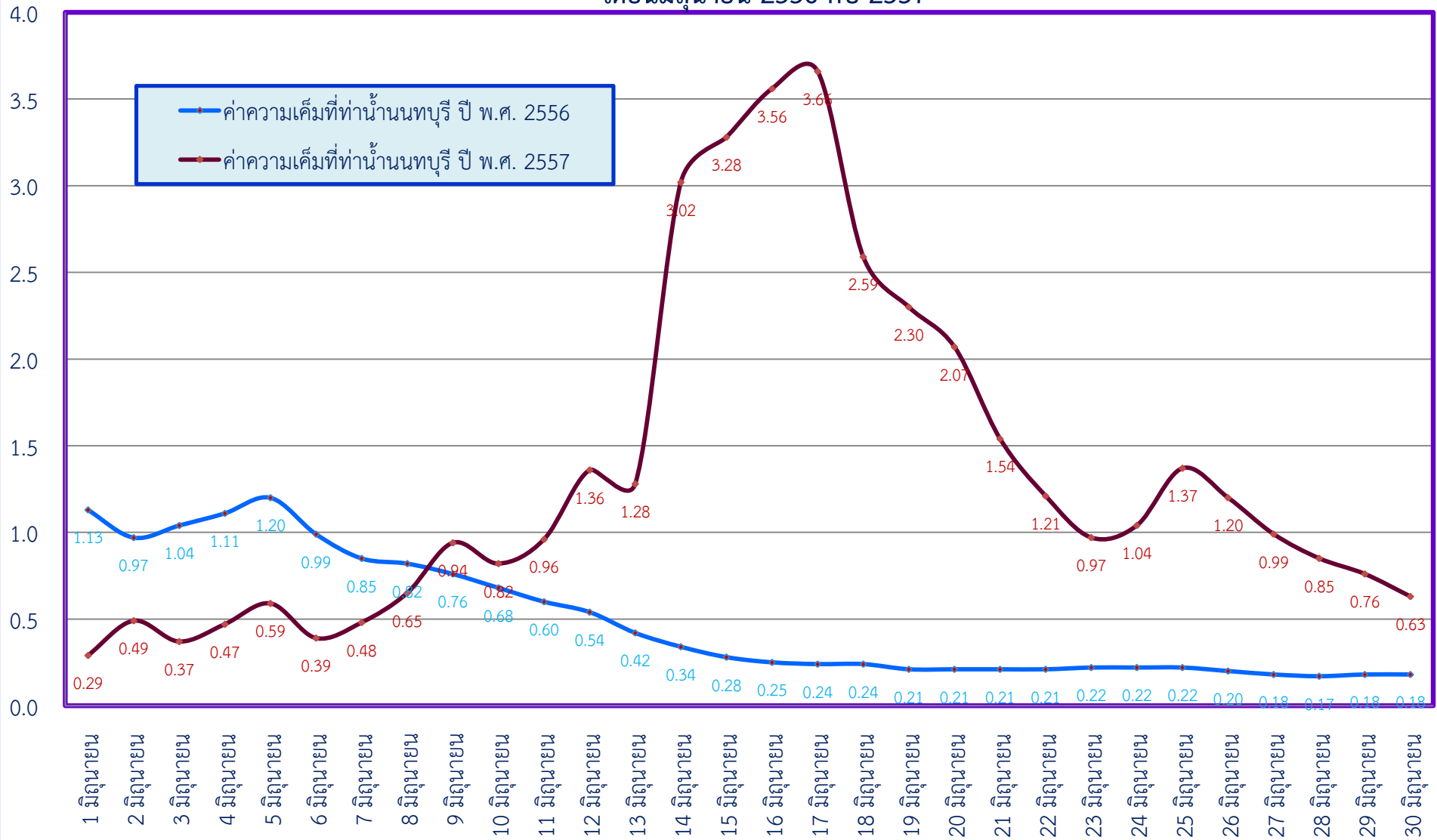
กราฟแสดงการเปรียบเทียบค่าความเค็มในแม่น้ำเจ้าพระยา ที่จุดตรวจวัดทำนายนนทบุรี เดือนมิถุนายน 2556 กับ 2557
